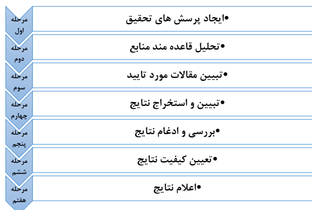
شکل ۱. مراحل فراترکیب
